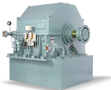
ID FAN FLUID COUPLING GEARBOX
